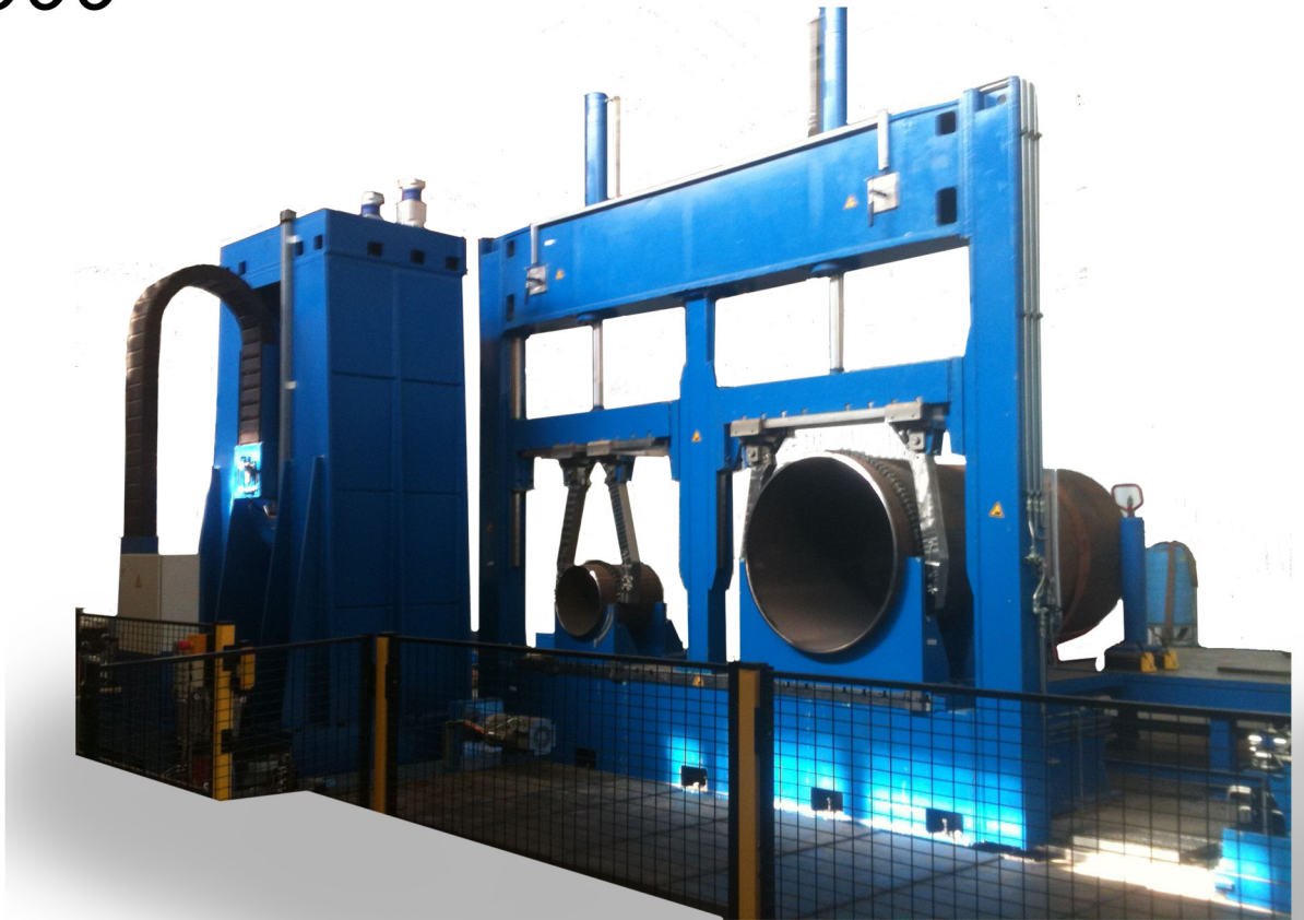
dazugehörige Spannstation
